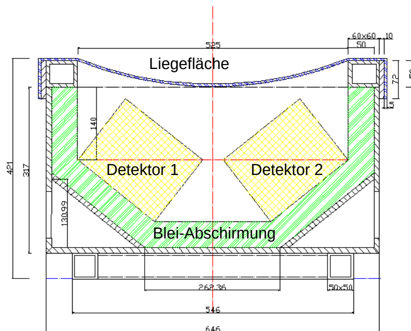
Abbildung 1-6: Schnitt durch den Ganzkörperzähler SM2
