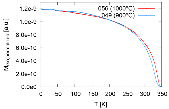
(d) SQUID of samples 049 (900 °C), 056 (1000 °C) FC
