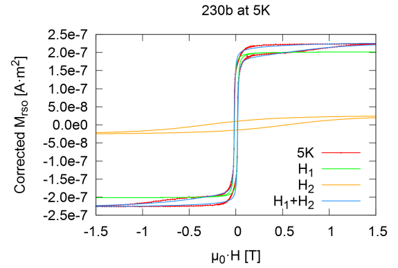
(d) Magnetization vs. field at 5K of 230b
