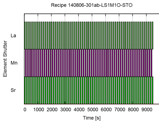
(d) MBE recipe 301ab
