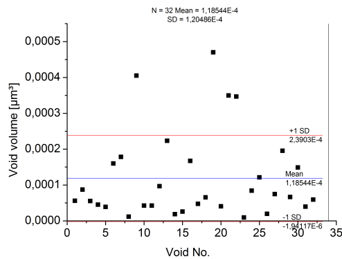
(b) Void volume
